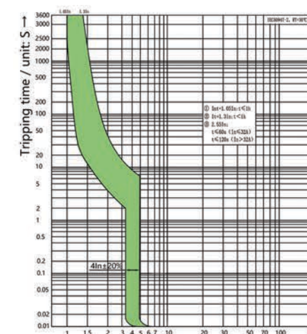
Krivka B 4I_n \pm 20\%
