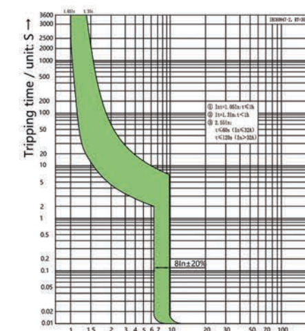
Krivka C 8I_n \pm 20\% Použitelný menovitý prúd \leq 63 A
